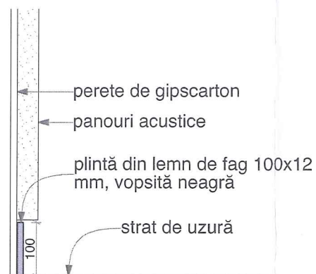
D-P-02.3 Detaliu plintă din lemn ascunsă, culoare neagră
