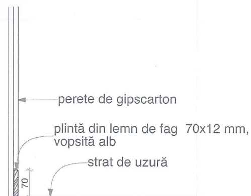
D-P-02.1 Detaliu plintă din lemn ascunsă, culoare albă
