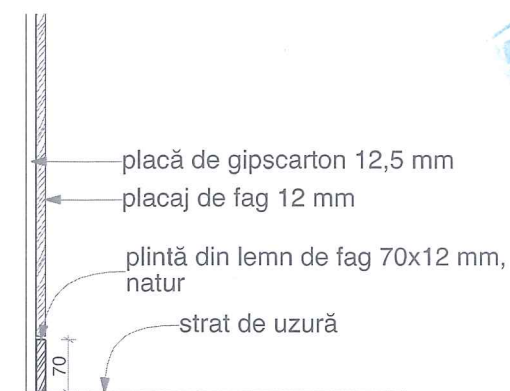
D-P-03 Detaliu plintă din lemn de fag, culoare natur
