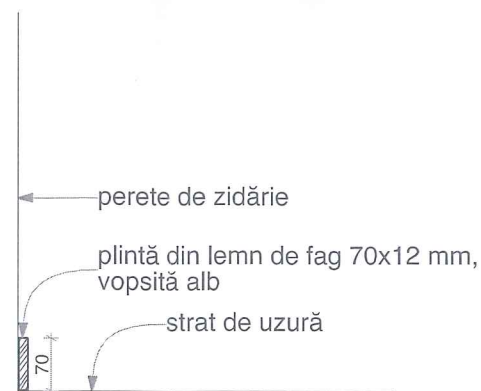
D-P-01.1 Detaliu plintă din lemn aplicată, culoare albă
