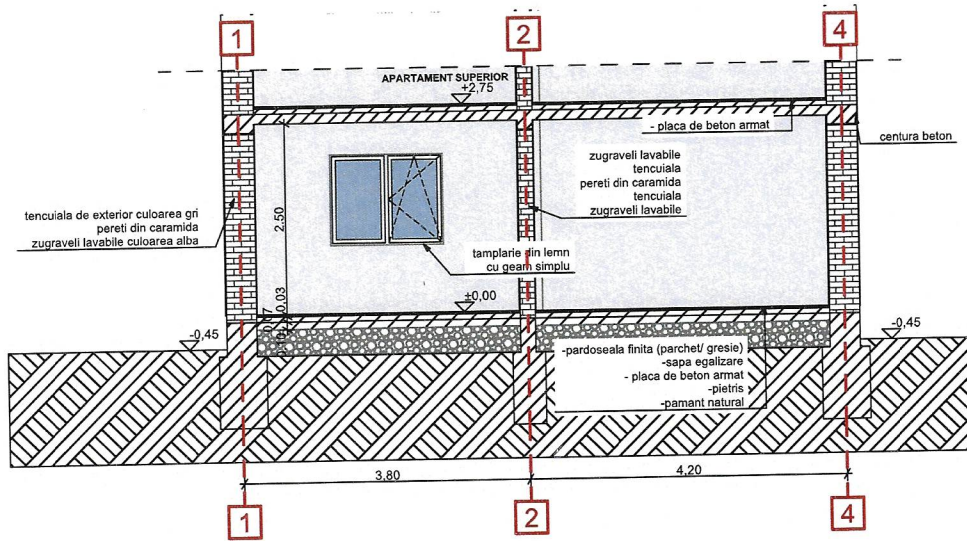
A SECTIUNE 1:100
