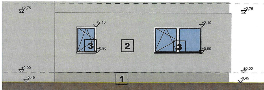
VEDERE EXTERIOR DREAPTA 1:100
