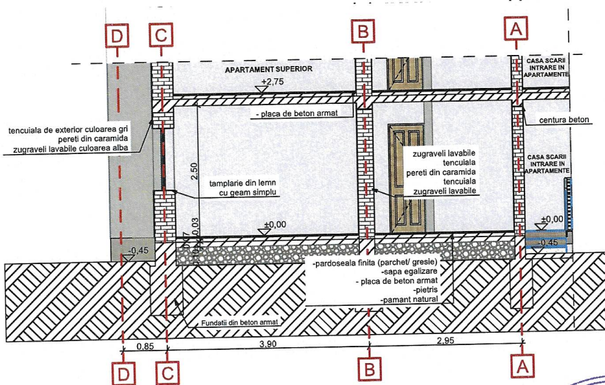
B SECTIUNE 1:100
