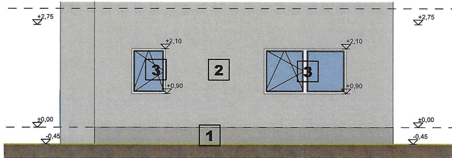
VEDERE EXTERIOR DREAPTA 1:100
