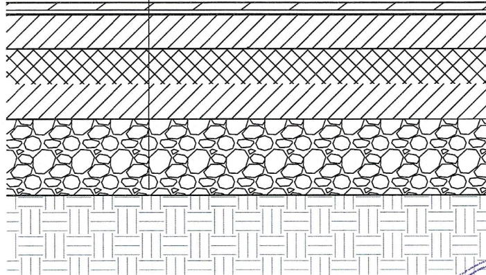
Detaliu parchet
