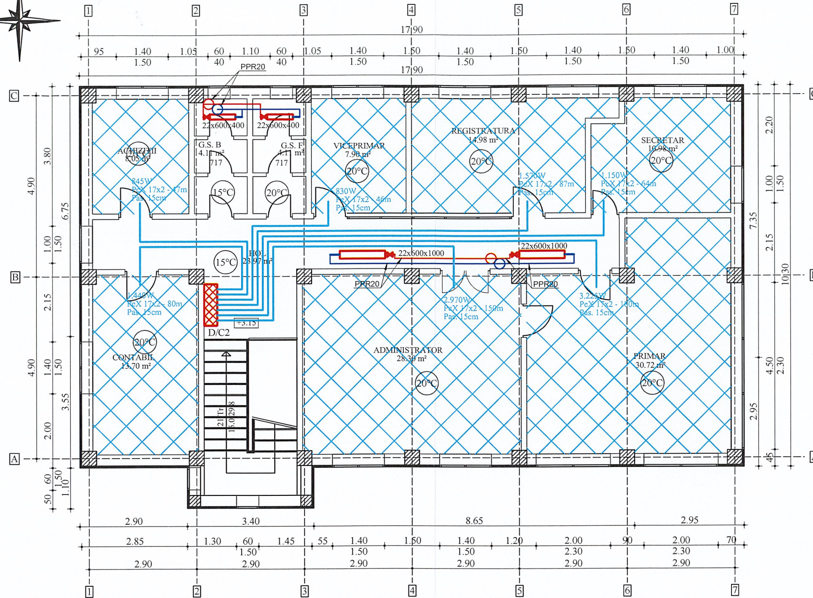
INSTALATII TERMICE PLAN ETAJ 1
