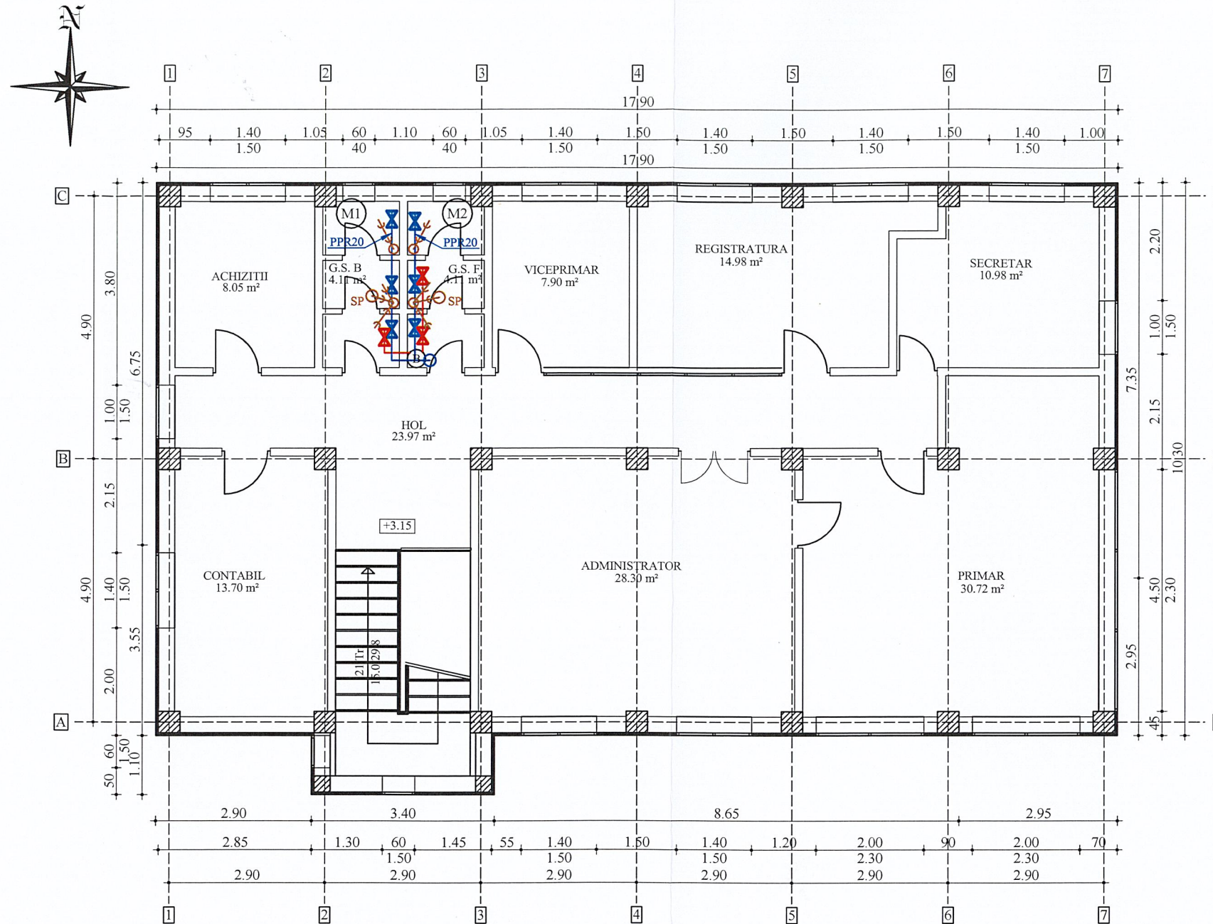
INSTALATII SANITARE PLAN ETAJ 1
