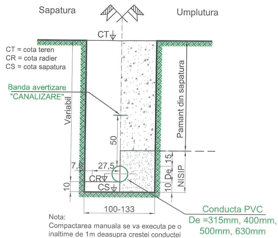
Detaliu pozare conducta din PVC De= 315mm, 400mm, 500mm, 630mm in zona drum asfaltat
