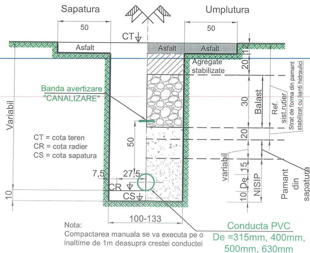
Detaliu pozare conducta din PVC De= 315mm, 400mm, 500mm, 630mm in zona drum asfaltat
