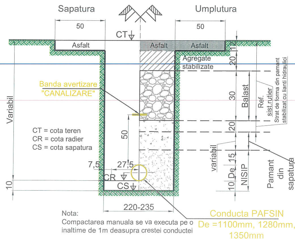
Detaliu pozare conducta din PAFSIN De= 1100mm, 1280mm, 1350mm in zona drum asfaltat
