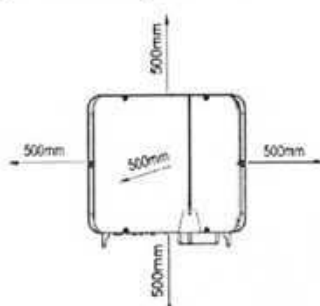
Figura 5.3 Distanțelor minime - În cazul unui singur inverter
