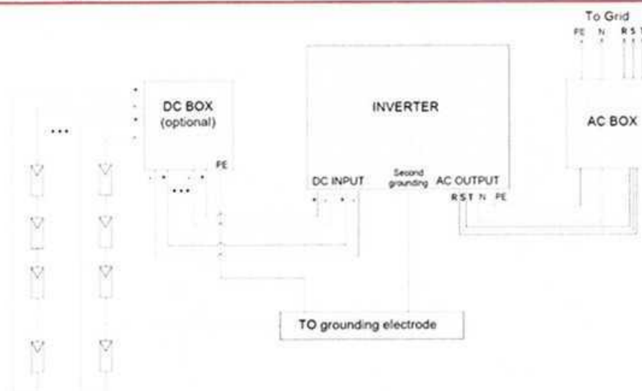
Fig.2.6 Schema de conexiune electrica inverter
