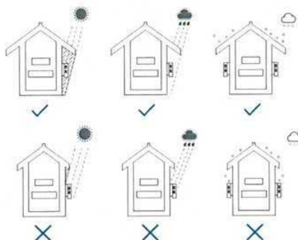
Figura 5.5 - Montaj optim propus
