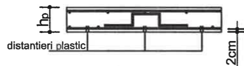
DETALIU DISTANȚIER planseu 15 cm scara 1:20
