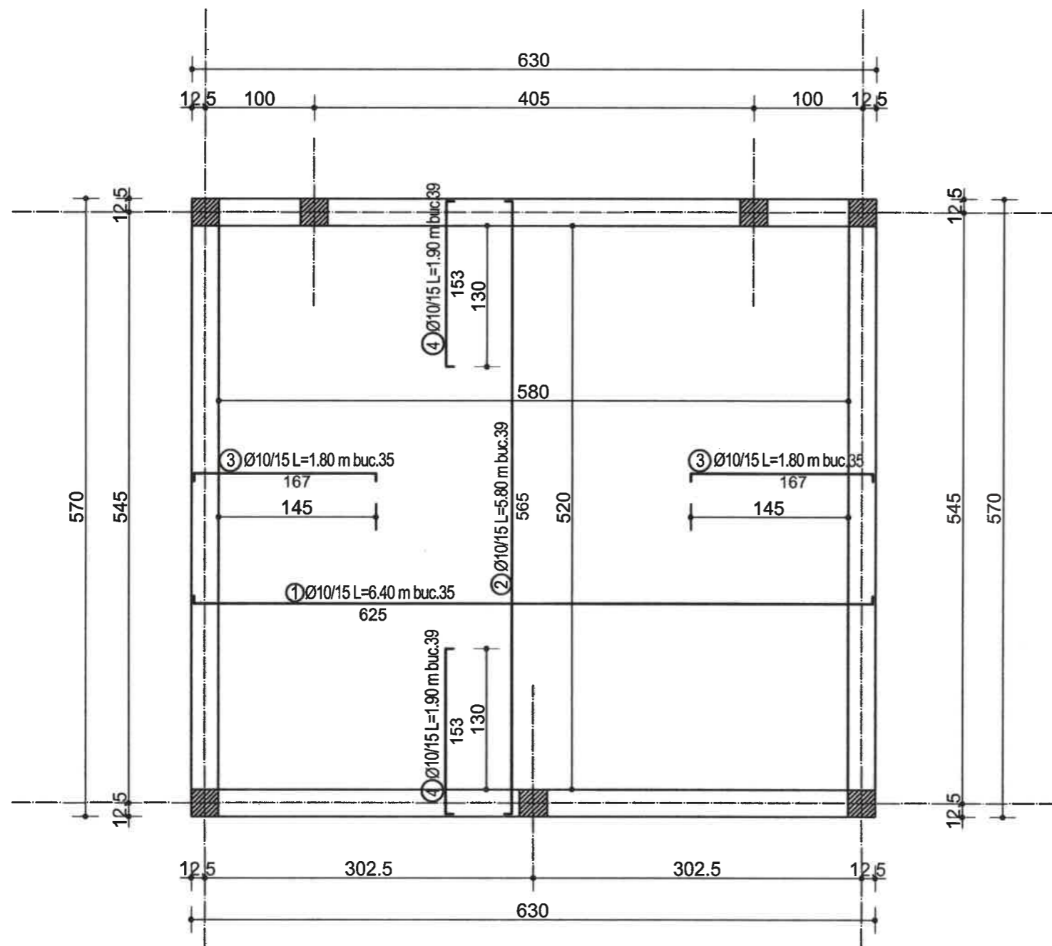
DETALIU DISTANȚIER MONTARE ARMATURI-PLANSEU 17CM scara 1:20
