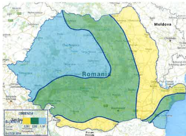
Fig. 3. Zonarea valorilor caracteristice ale încărcării din zapada pe sol s_k , kN/m^2 , pentru altitudini A \leq 1000 m
