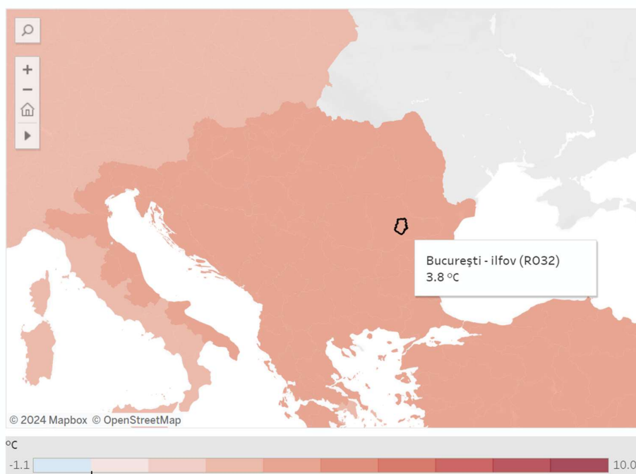
Figure 5 Modificarea proiectată a mediei lunare a temperaturii medii zilnice in perioada verii
