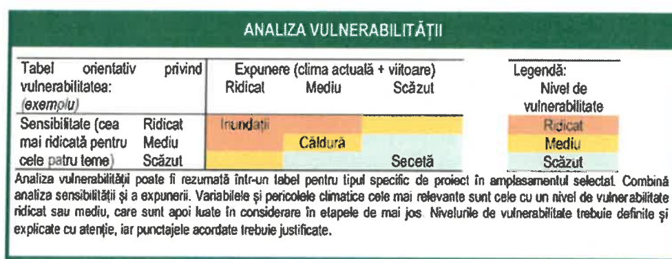
Figure 17 Analiza vulnerabilității
