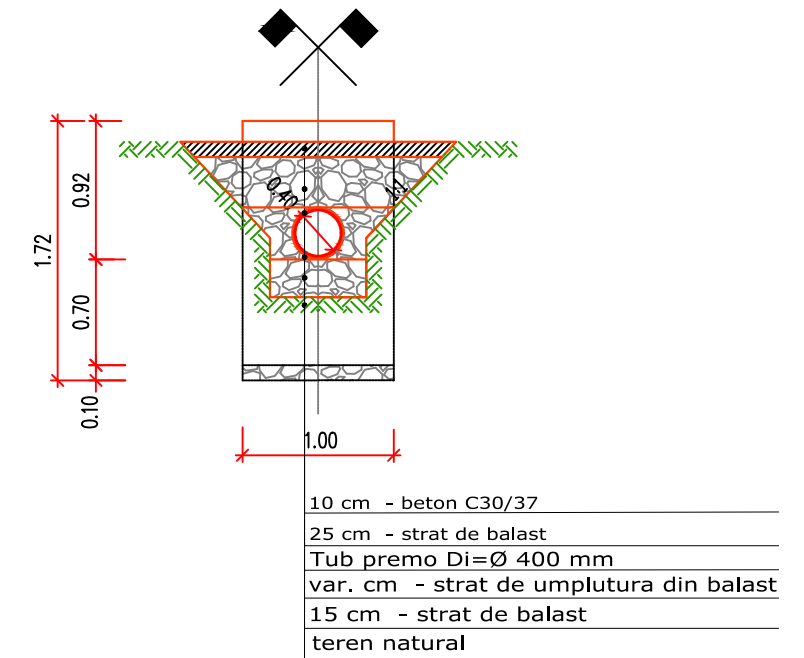
SECȚIUNE B - B
