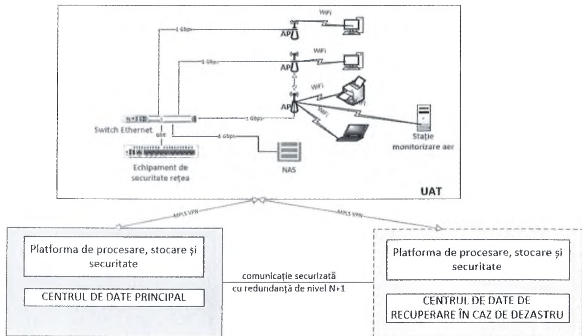
Figura 2: Arhitectura fizică a PISE
