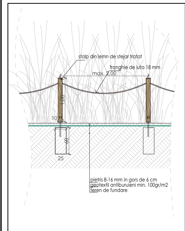
Sectiune 2 1:50
