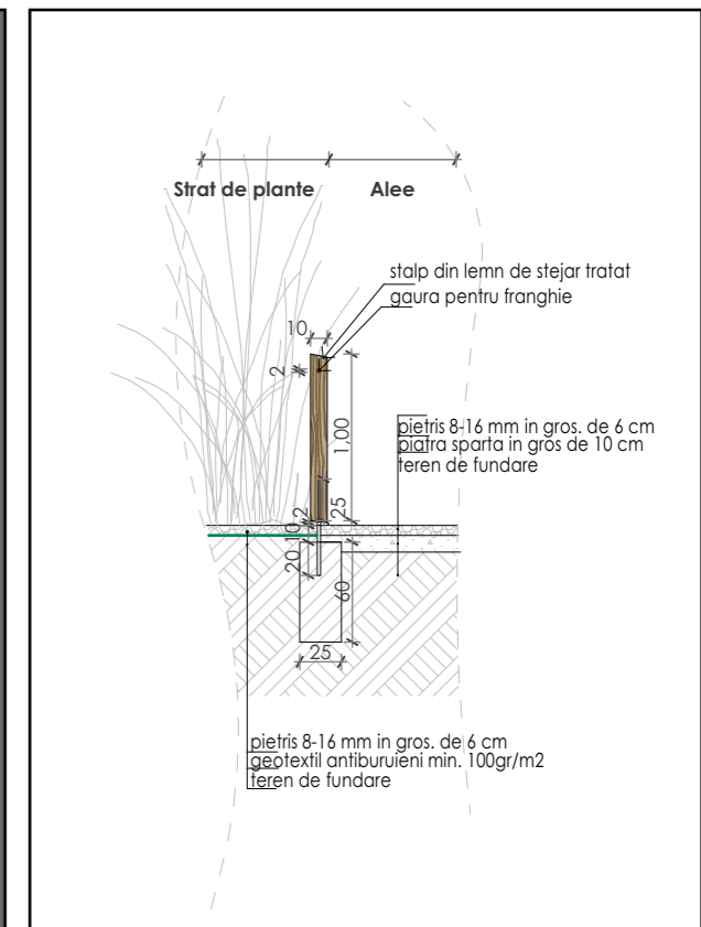
Sectiune 1 1:50
